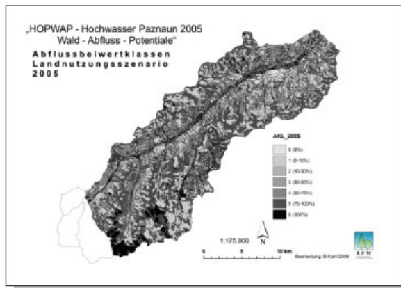
Abb. 4: Oberflächenabflussklassen für das Landnutzungsszenario 2005. Fig. 4: Surface runoff classes for scenario land use 2005.
